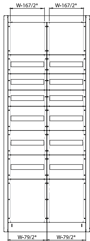
פנלים (חלוקה ל-2 שדות)
