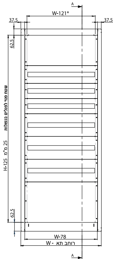
פנלים (חלוקה לשדה 1)
