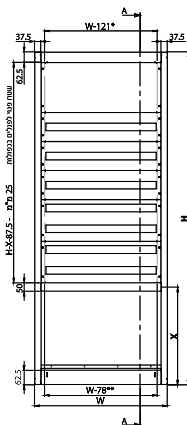
פנלים (חלוקה לשדה 1)
