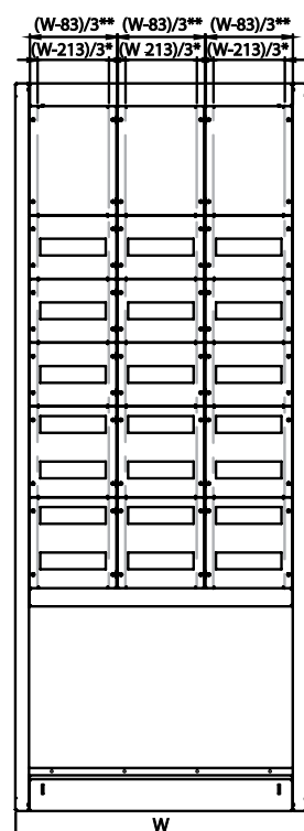
פנלים (חלוקה ל-3 שדות)
