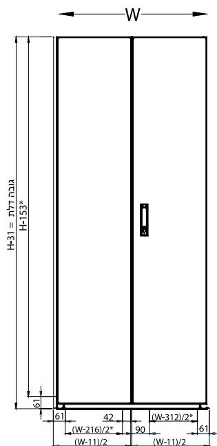
דלת כפולה עם מנעול מרכזי
