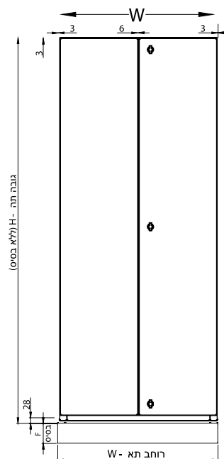
מכנה ארון עם דלת כפולה
