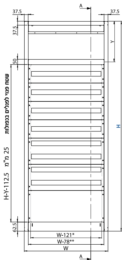
פנלים (חלוקה לשדה 1)
