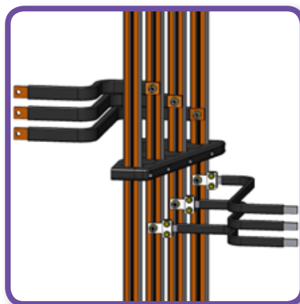
גישה מלאה לחיבור מוליכים לפסי הצבירה משני הצדדים
