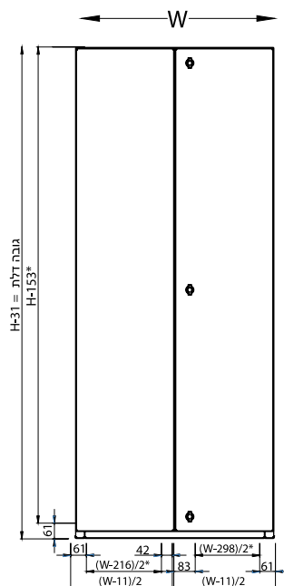
דלת כפולה עם מנעול פרפר
